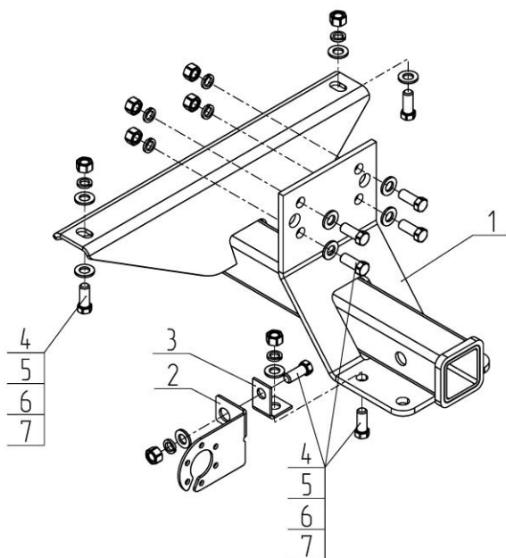
Рис.1 Установка на автомобиль
