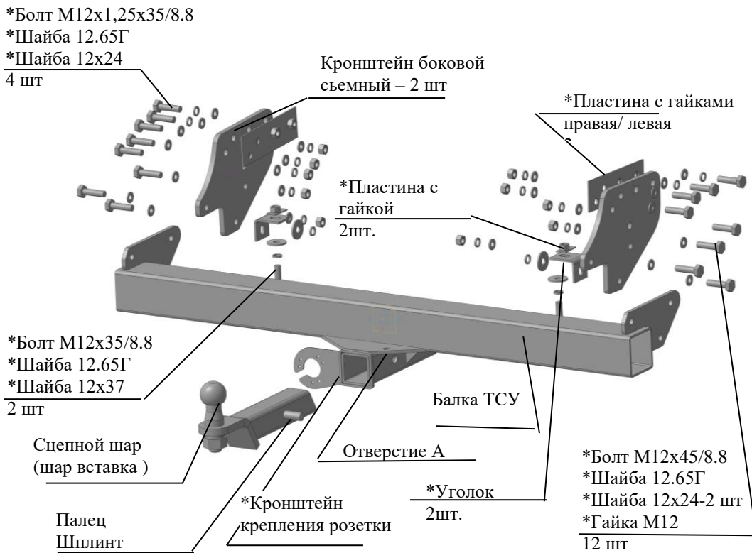
Рис.1 Тягово-цепное устройство 7113.
