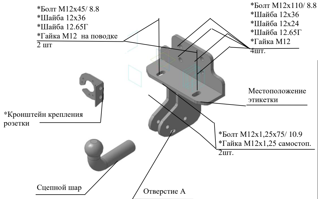
Рис.1 Тягово-сцепное устройство 7821.
