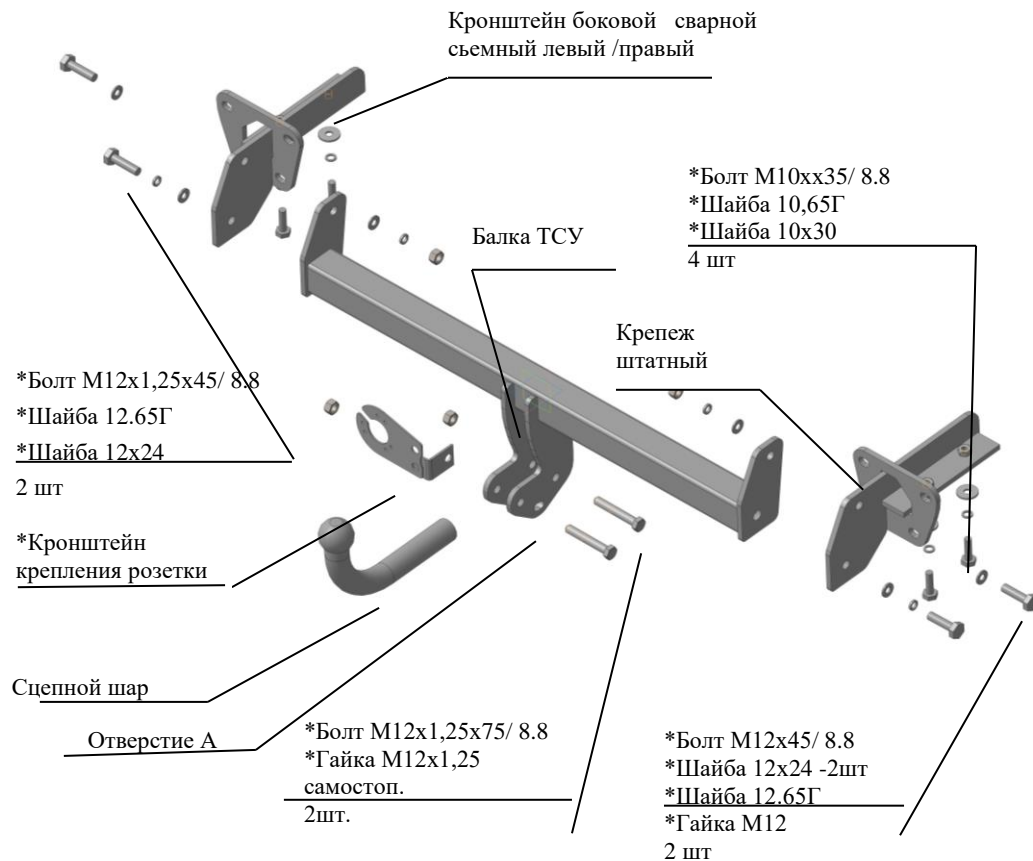
Рис.1 Тягово-сцепное устройство 8520 .
