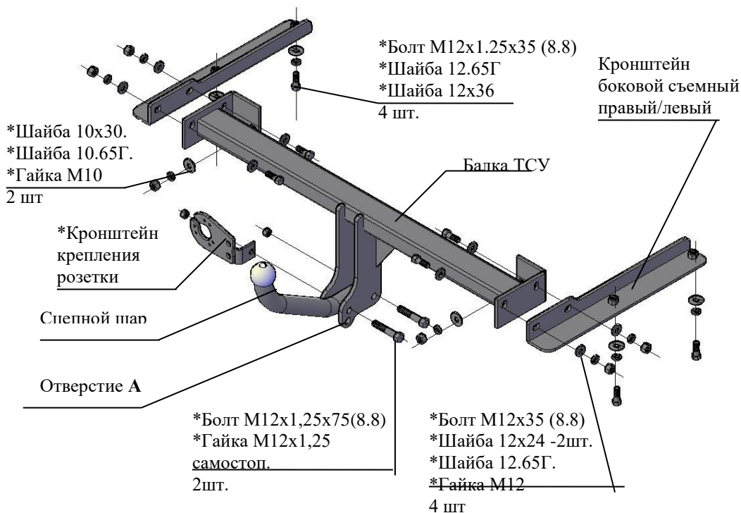
Рис.1 Тягово-сцепное устройство 9931
